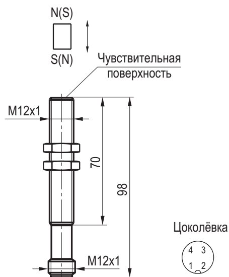
Габаритный чертеж
