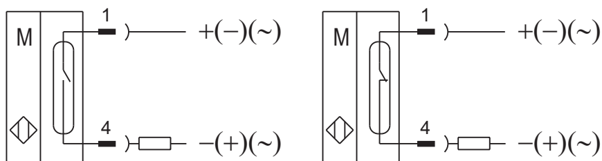
Схемы подключения нагрузки
